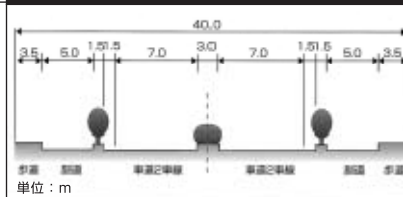
道路幅員構成[副道設置区間]
