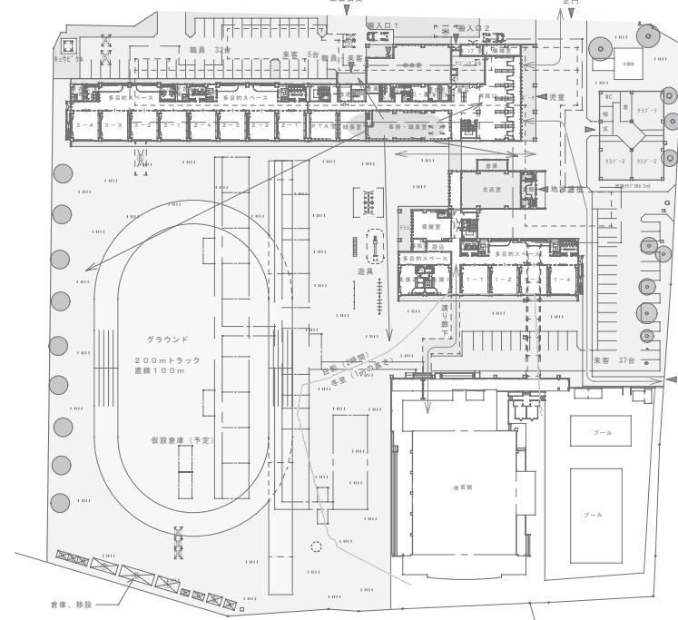
鏡石町立第一小学校完成配置図
